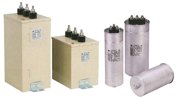
UV乾燥機用電容器
