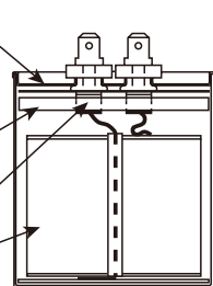
正常使用時(動作前) Normal Condition
